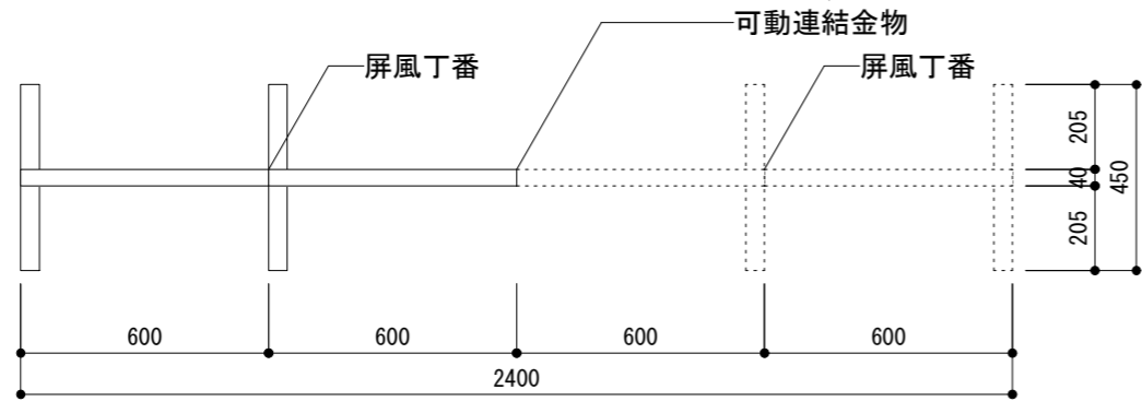
上面図
