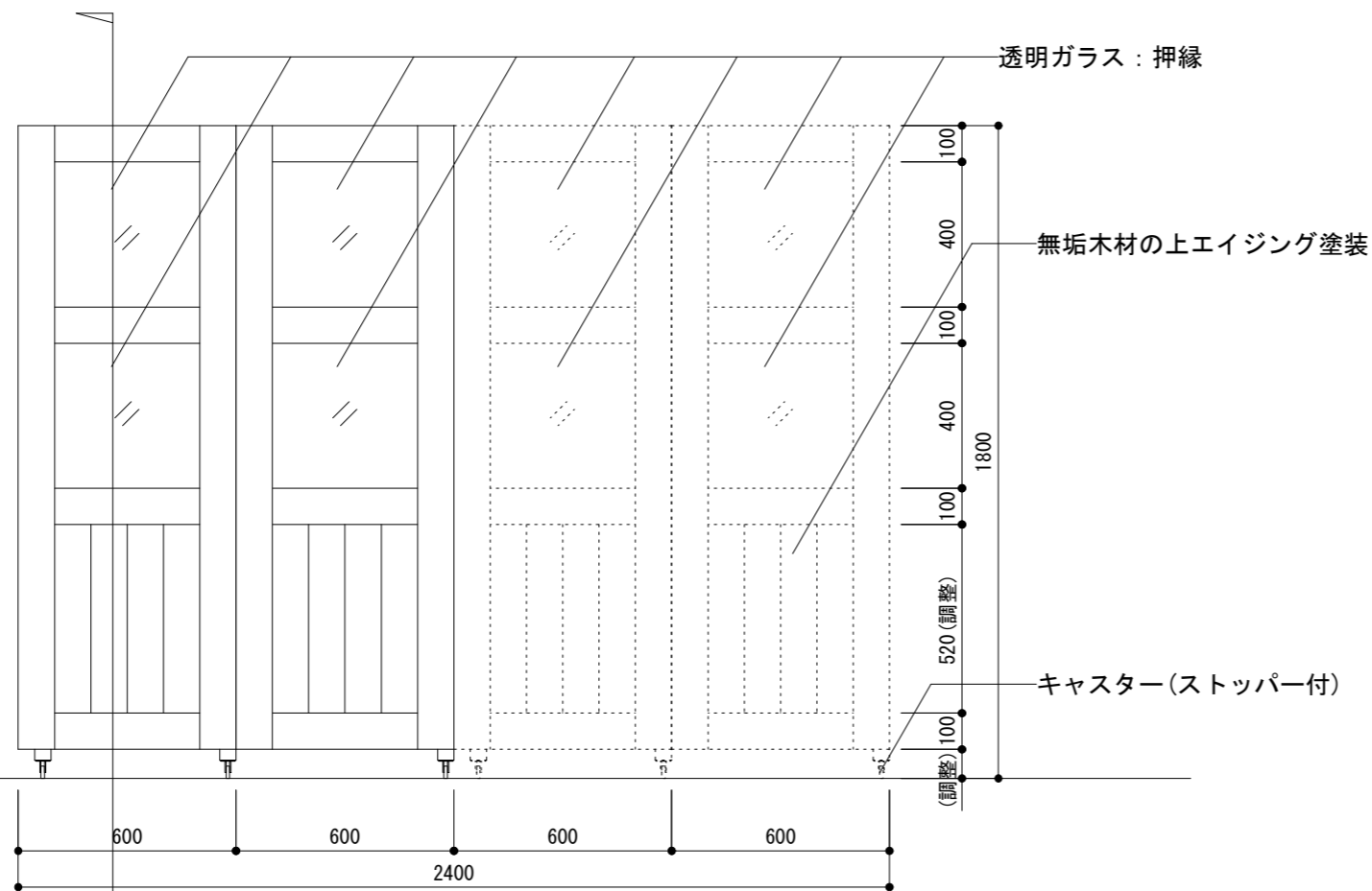
正面図
