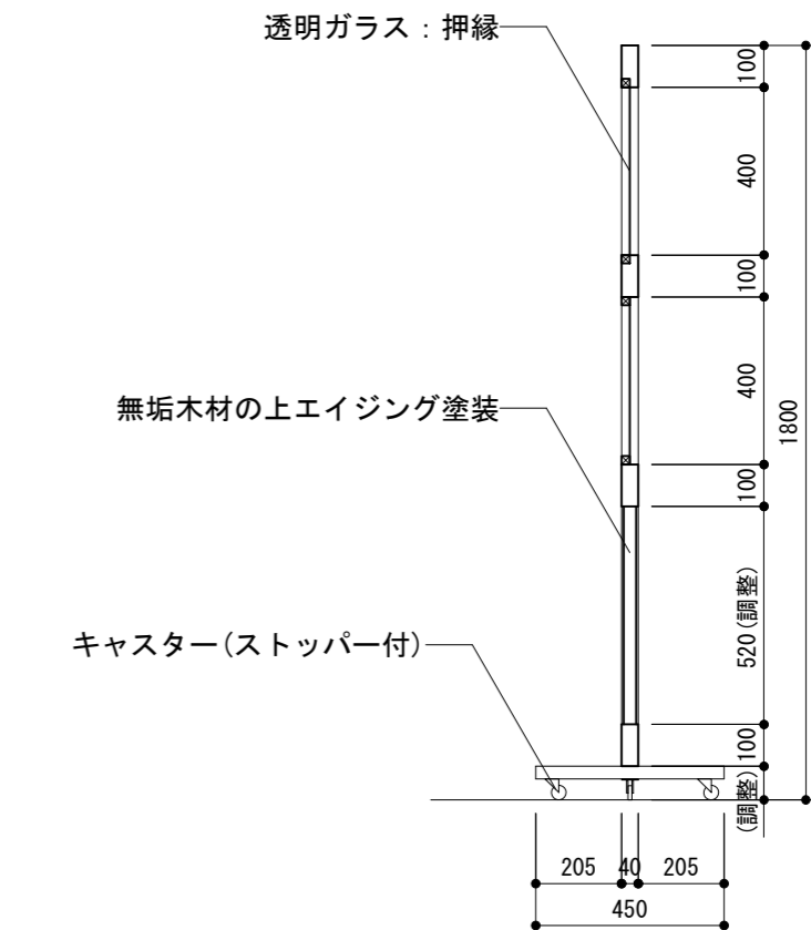
断面図
