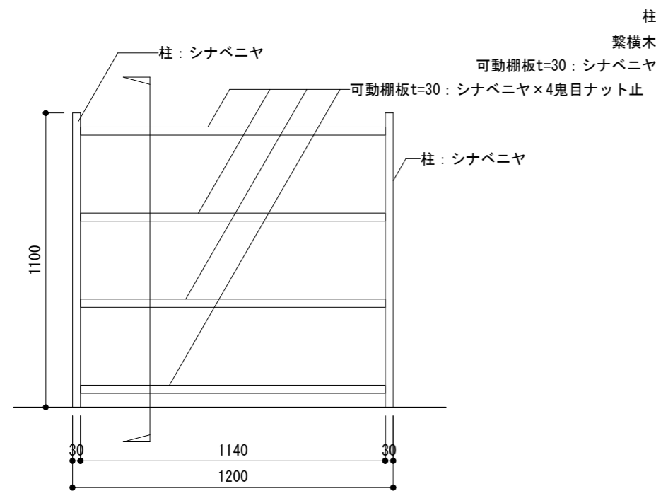
正面図
