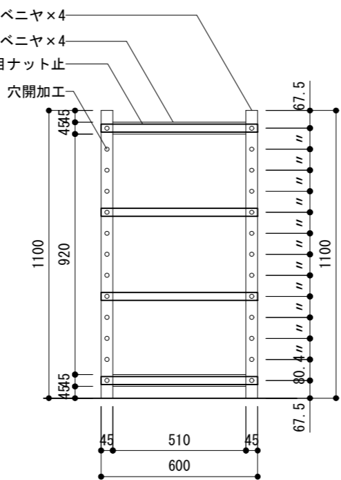
断面図
